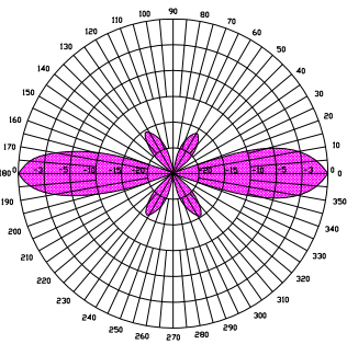
垂直方向图
